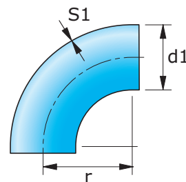
Codos prensados
